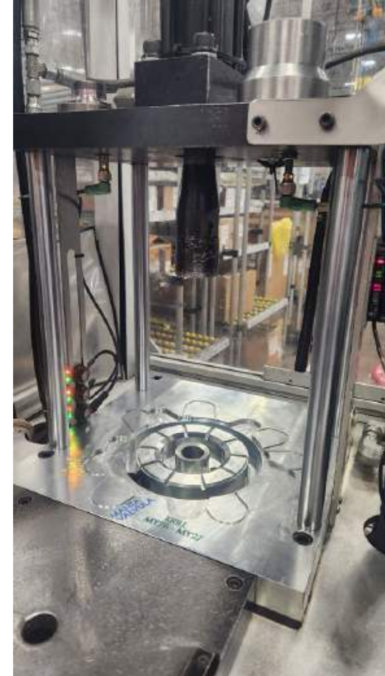
PRENSA DE INSERCIÓN DE BALERO
