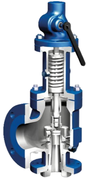
Válvulas de seguridad ANSI Bridadas y Roscadas
