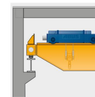
Conexión de viga principal estándar en combinación con polipasto de altura rebajada.
