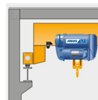
Versión sobreelevada, variante 5
