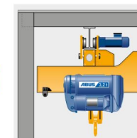
Conexión a viga principal de serie, variante 1 con viga ensanchada (voladizo variable para maximizar el desplazamiento del carro)
