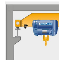
Conexión a viga principal de serie, variante 3
