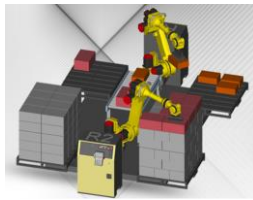
RoboGuide Fanuc.
