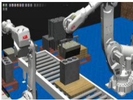
RoboStudio ABB.
