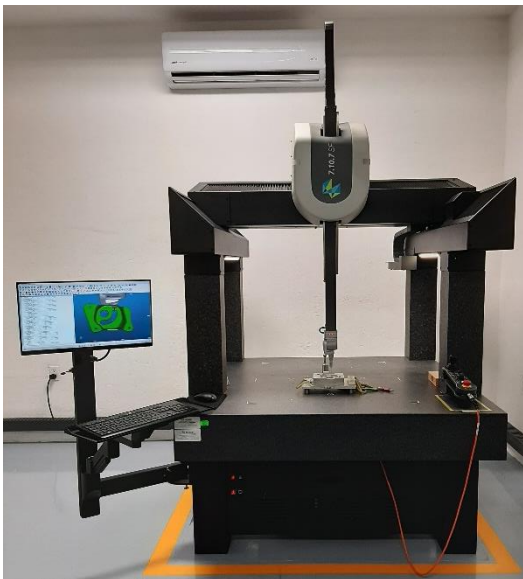
CMM Hexagon 7.10.7 SF
